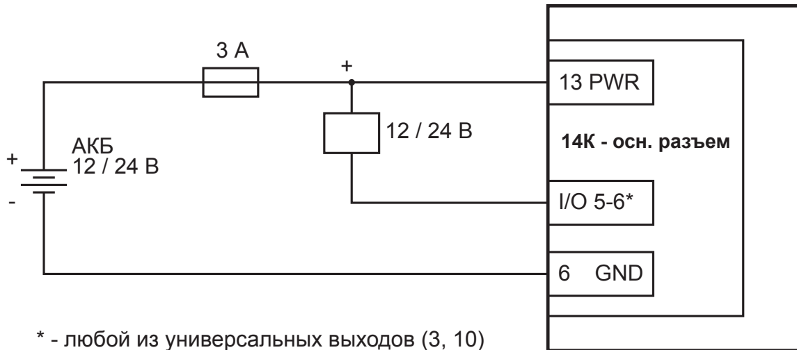
Рис. 3.11. Схема подключения реле к выходу (12 В)
