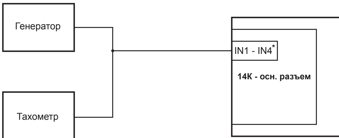
Рис. 3.5. Схема подключения тахометра
