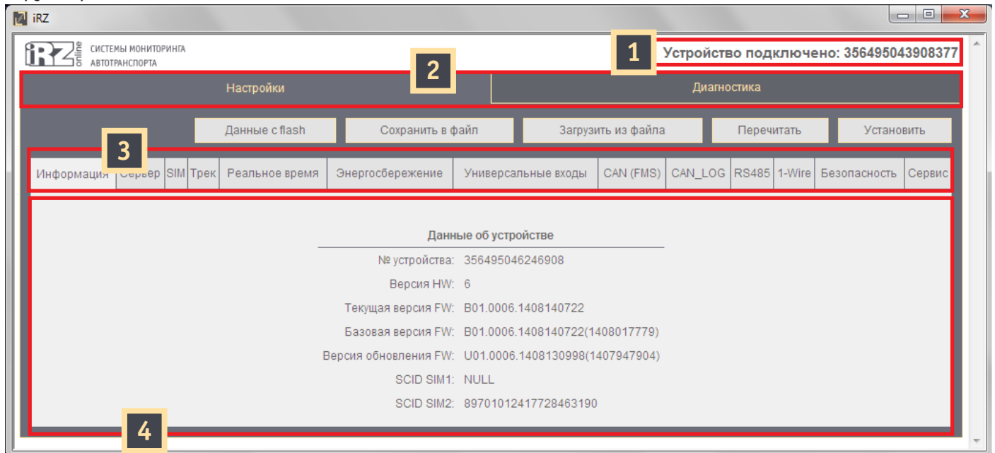
Рис. 4.1. Программа-конфигуратор
